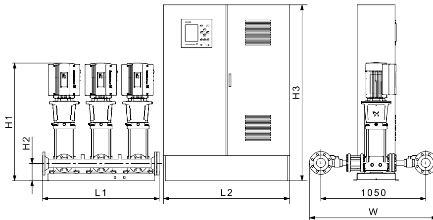
Рис. 59 Размерная схема установки повышения давления Hydro MPC со шкафом управления, смонтированным на полу (исполнение C). Установка повышения давления приведена в качестве примера. Входящие в поставку насосы могут отличаться от показанных на схеме.
