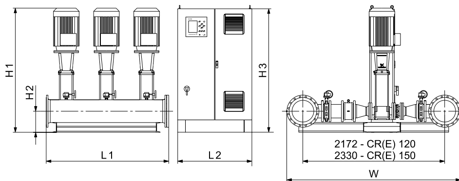
Рис. 63 Размерная схема установки повышения давления Hydro MPC со шкафом управления, смонтированным на отдельной раме-основании (исполнение D). Установка повышения давления приведена в качестве примера. Входящие в поставку насосы могут отличаться от показанных на схеме.
