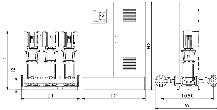
Рис. 42 Размерная схема установки повышения давления Hydro MPC со шкафом управления, смонтированным на полу (исполнение С). Установка повышения давления приведена в качестве примера. Входящие в поставку насосы могут отличаться от показанных на схеме.
