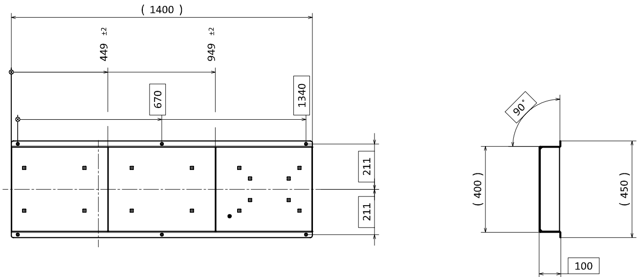
Рис. 92 Плита-основание
