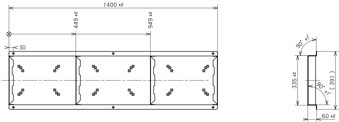
Рис. 91 Плита-основание
